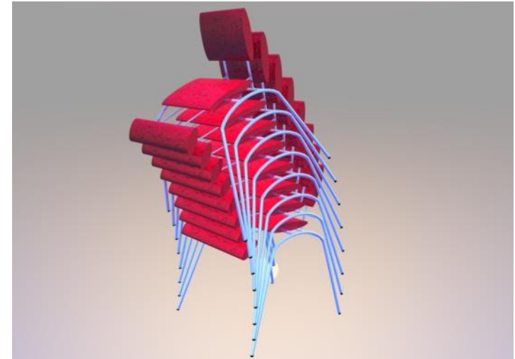
スタッキング検討図 3DCG
